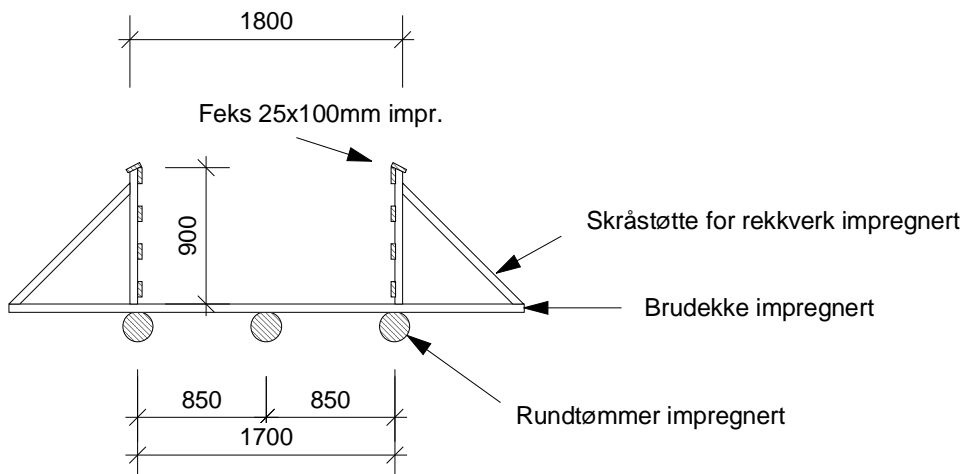
Snitt M 1 : 50
