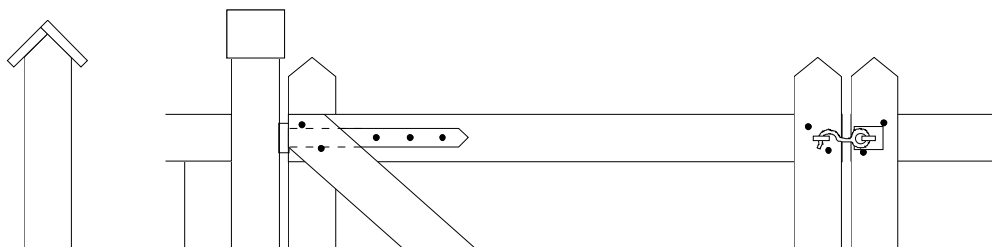
Alternativ detaljutføring av stolper
